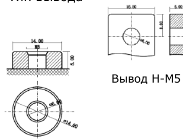
Вывод V-M6
